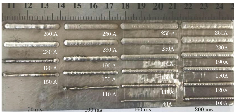
图 3 不同冷焊电流和时间下 TIG 冷焊熔敷焊道的表面形貌
