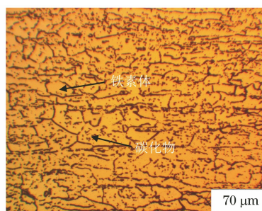
图 1 1Cr17 不锈钢的显微组织
