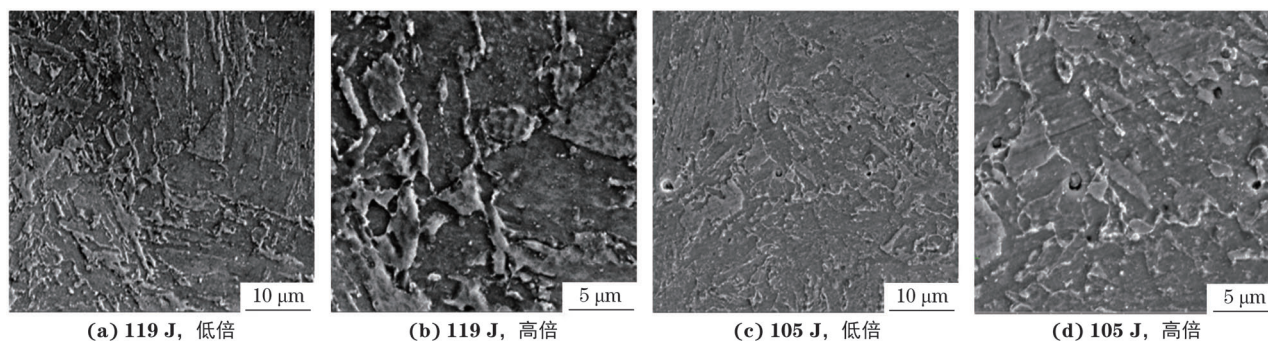
图 5 55 °C·h -1 焊后热处理冷却速率下不同冲击吸收能量的焊缝金属裂纹源附近的微观形貌 (道间温度 250 °C)
