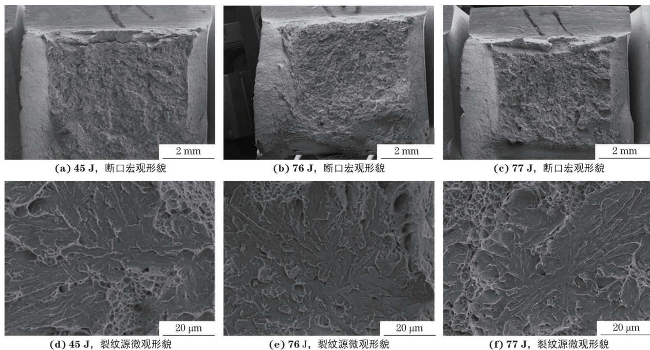
图 4 300 °C 道间温度和约 20 °C·h -1 焊后热处理冷却速率下不同冲击吸收能量的焊缝金属断口宏观形貌与裂纹源微观形貌
